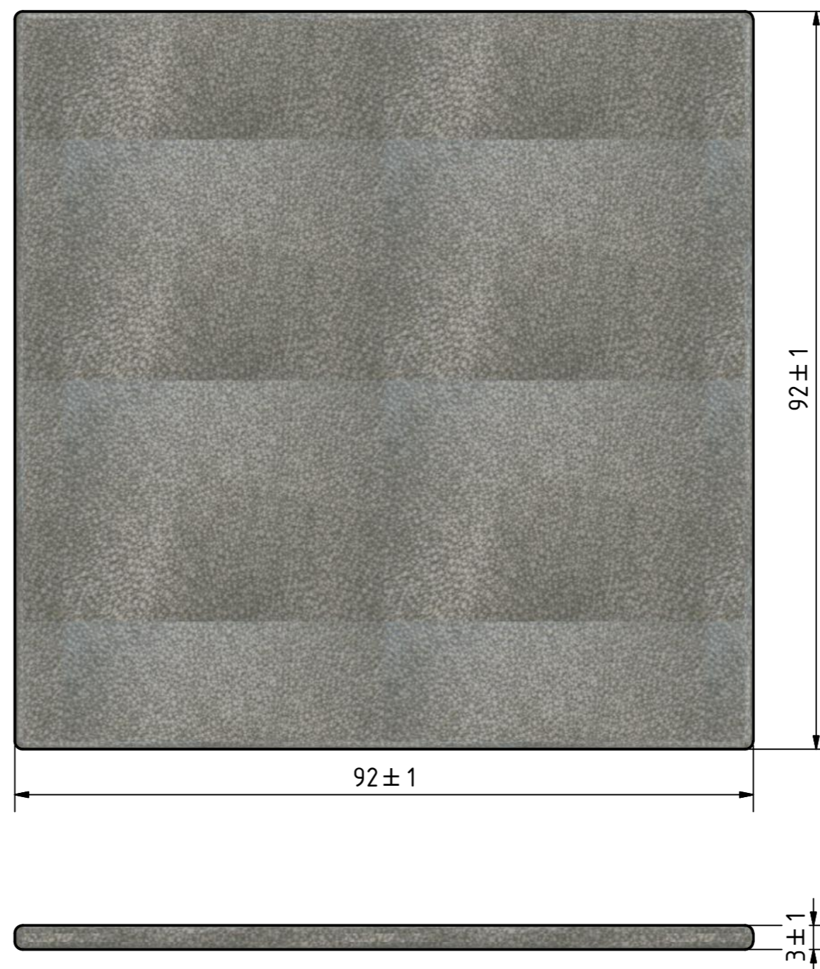
Filtereinsatz
