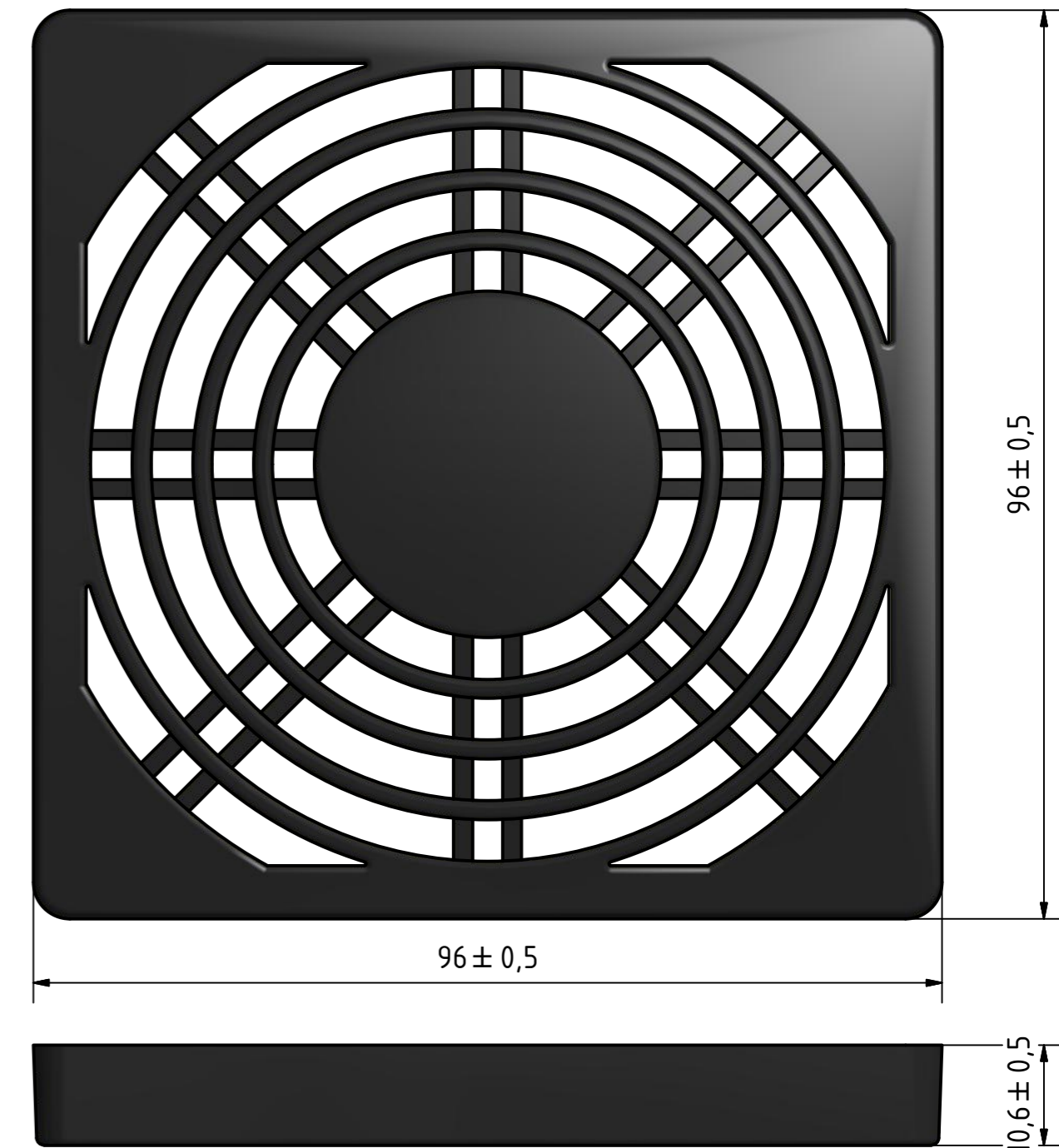
Außengitter
